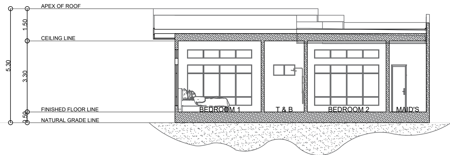
1 CROSS SECTION A3 A5 SCALE 1 : 100 M.
