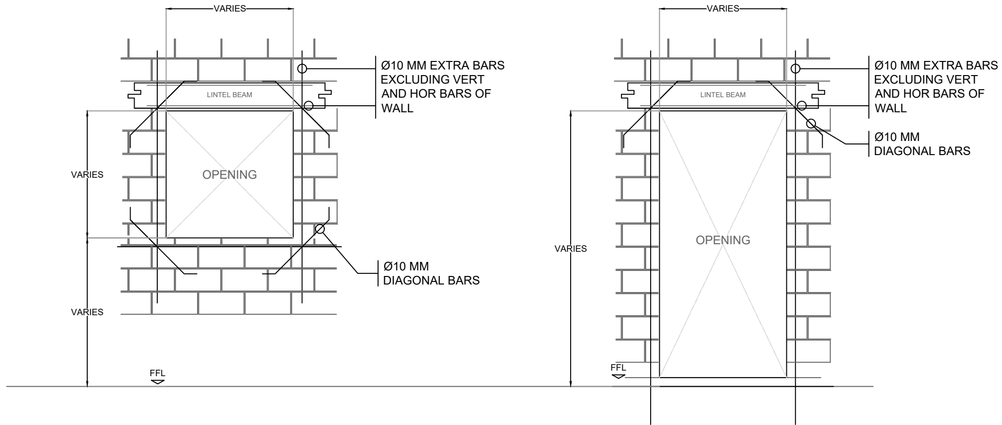
4 DOOR & WINDOW OPENINGS SCALE 1 : 30 M.
