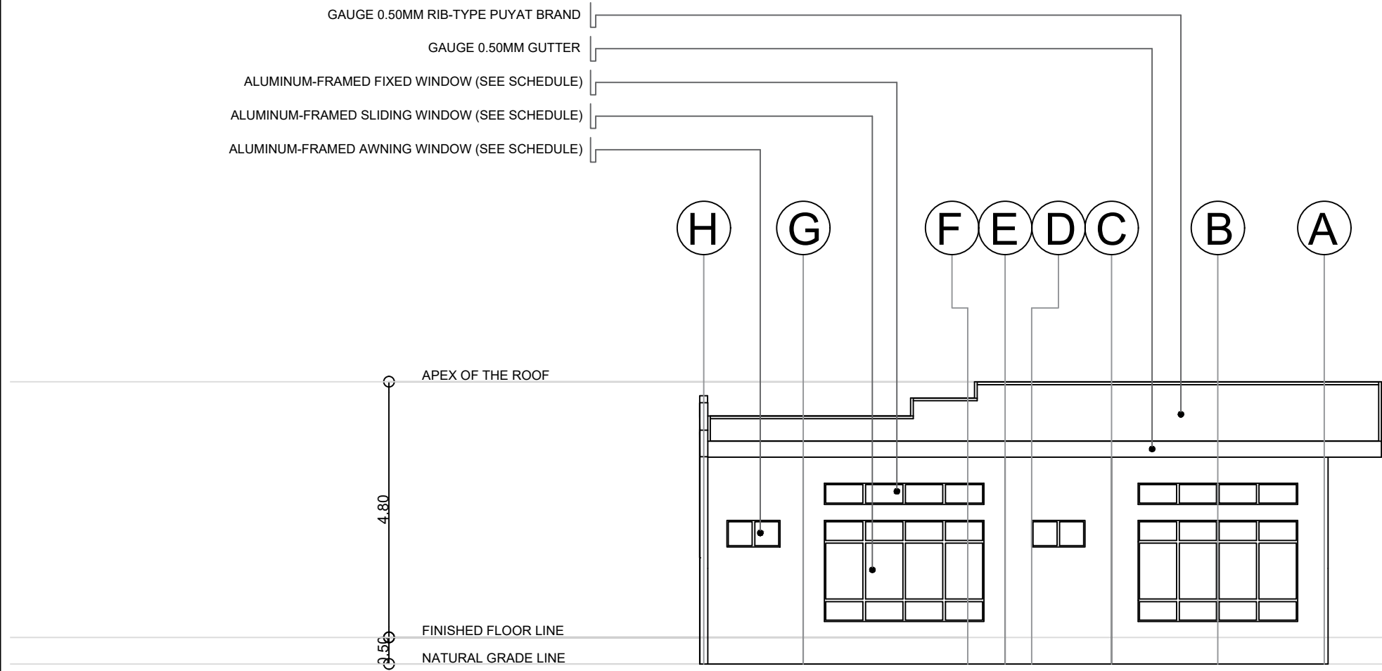
3 REAR ELEVATION A4 A5 SCALE 1 : 100 M.
