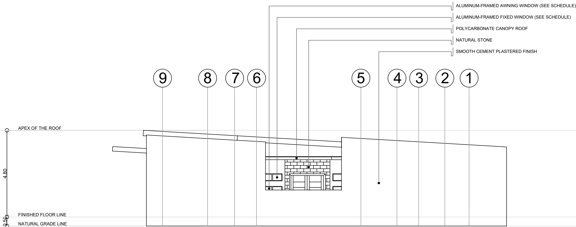
2 RIGHT SIDE ELEVATION A4 A5 SCALE 1 : 100 M.
