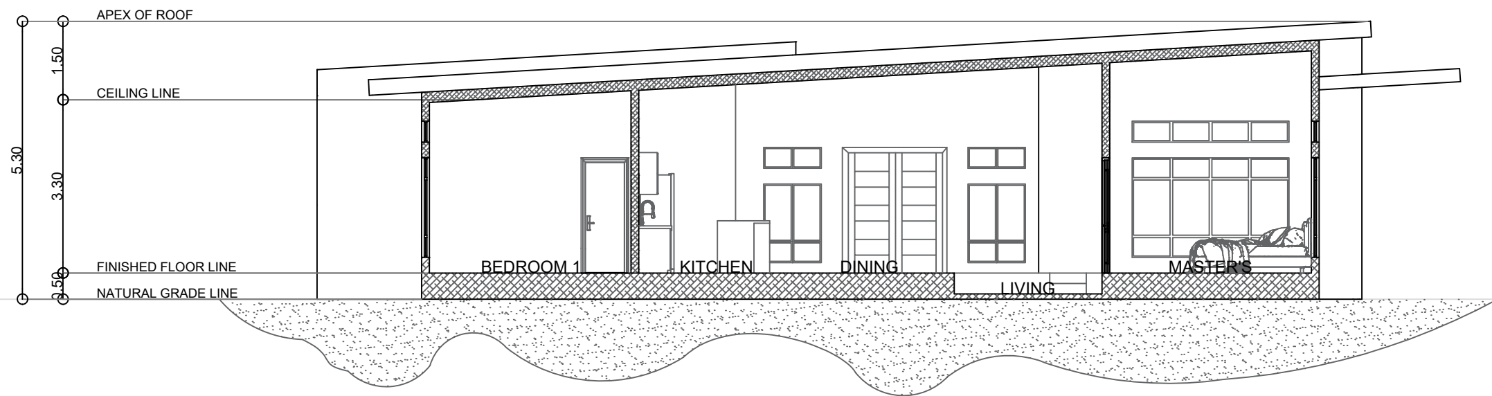
2 LONGITUDINAL SECTION A3 A5 SCALE 1 : 100 M.
