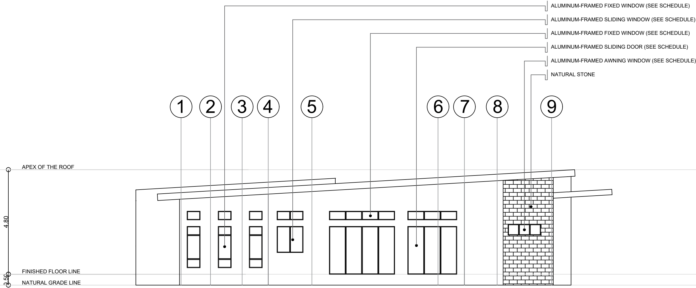
4 LEFT SIDE ELEVATION A4 A5 SCALE 1 : 100 M.
