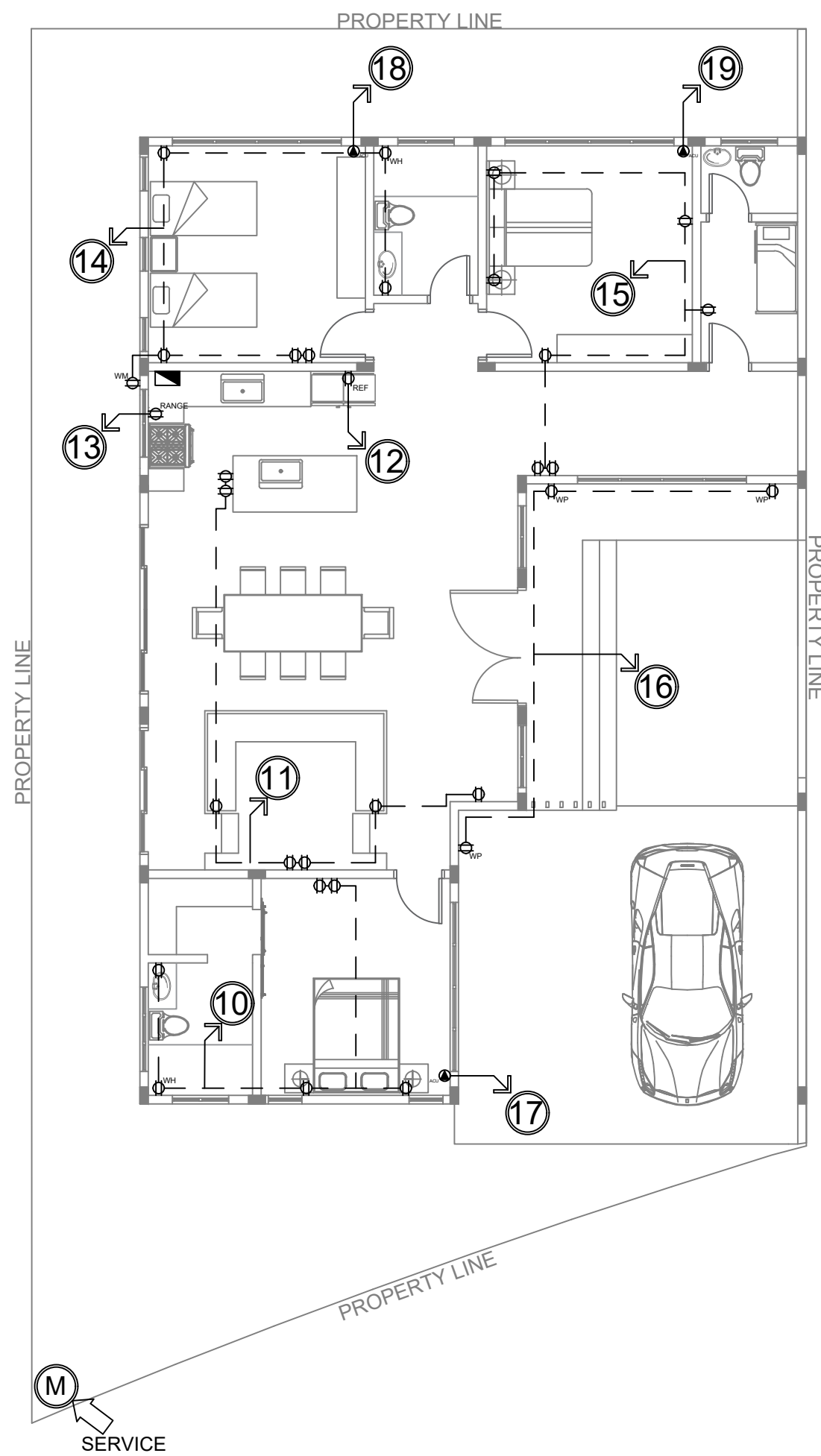
2 POWER LAYOUT E1 E1 SCALE 1 : 100 M.
