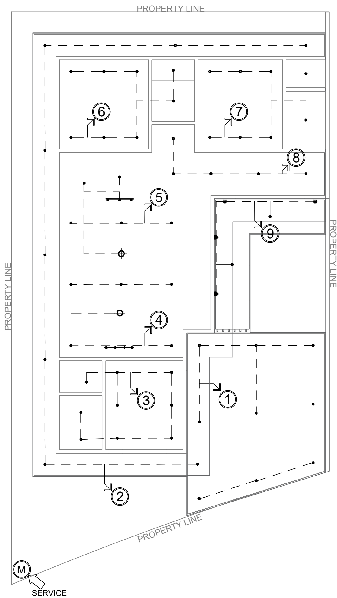
1 LIGHTING LAYOUT E1 E1 SCALE 1 : 100 M.
