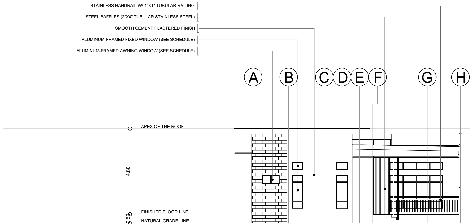
1 FRONT ELEVATION A4 A5 SCALE 1 : 100 M.
