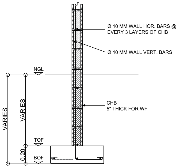
5 WF DETAIL SCALE 1 : 20 M.
